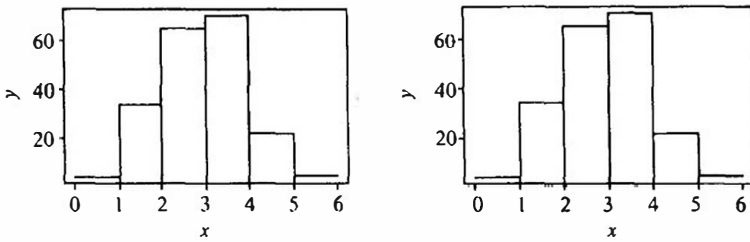
图 1.1 直方图
