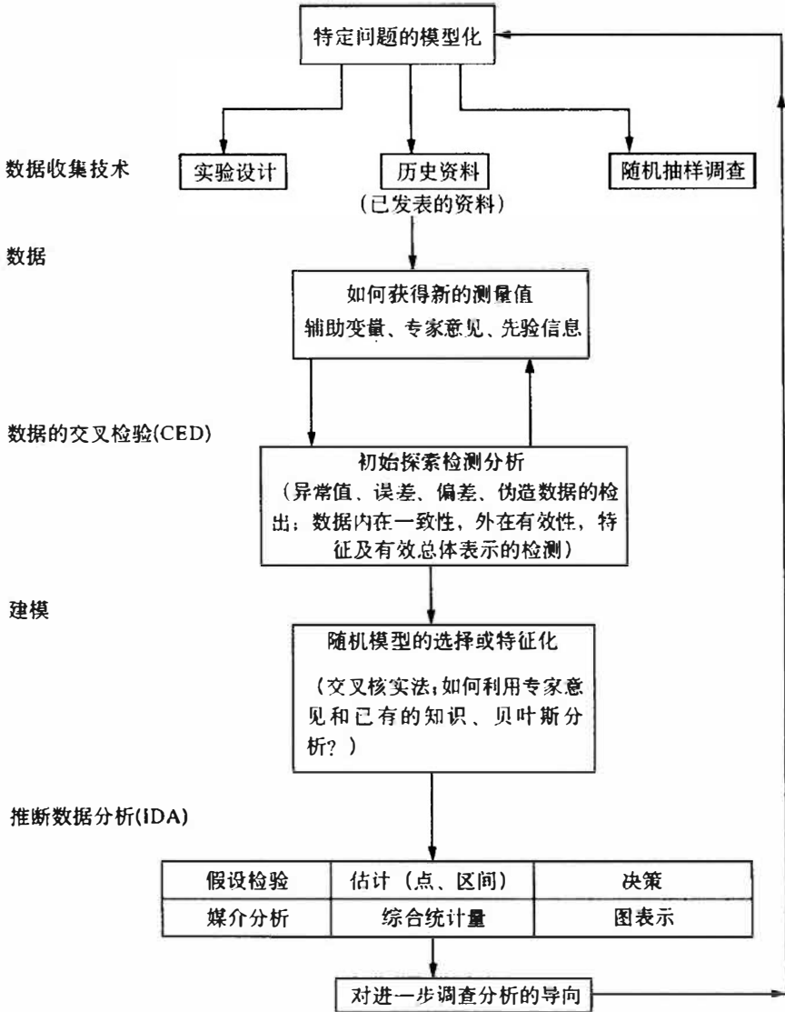
图 3.1 统计分析的步骤
