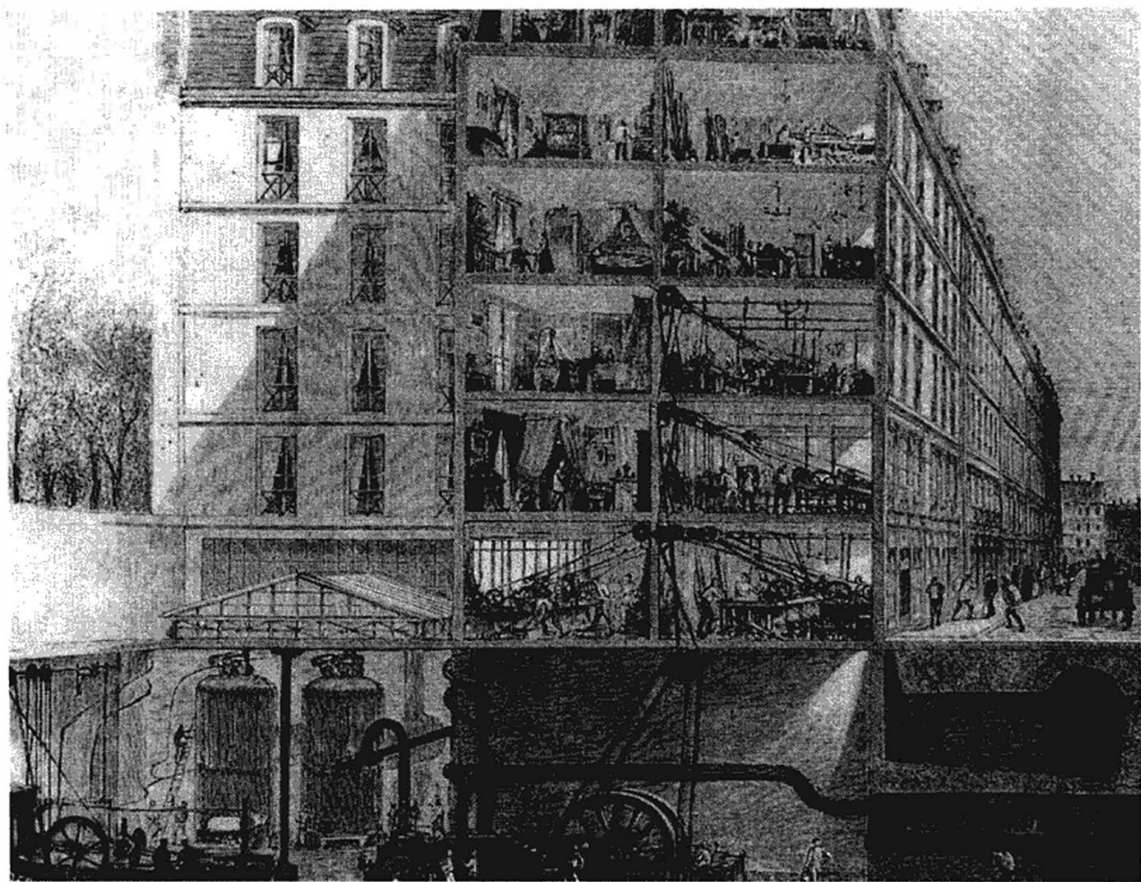
FIGURE-061 蒸汽引擎的集体使用成了这段时期巴黎的产业特征。这张 1872 年的设计图说明这个系统——通过地下室的蒸汽引擎来运作，并将动力分配到上面的楼层——如何允许整栋建筑物由不同行业来使用。
